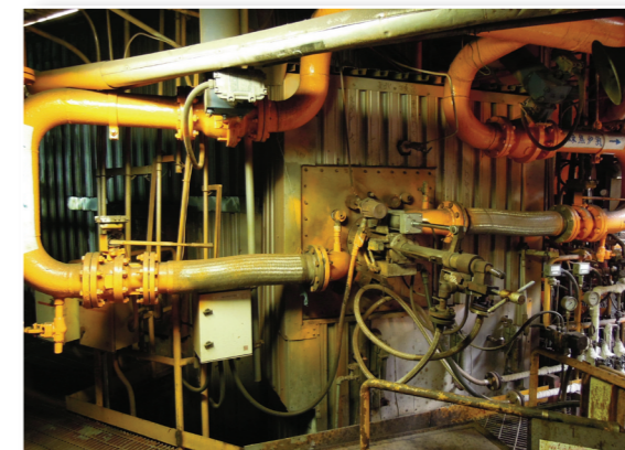
鍋爐輔助燃料焦爐氣燃燒器及管線
