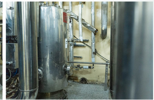
殺菌釜設備優化，增設儲水桶
