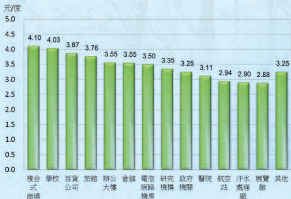
圖 5. 單位用電度數平均電價指標 (元 / 度)
