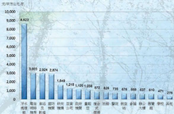
圖 4. 單位面積能源費用指標 (元 / 平方公尺 · 年)
