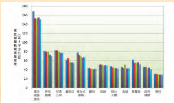
圖 8. 近五年單位面積耗電需量密度變化
